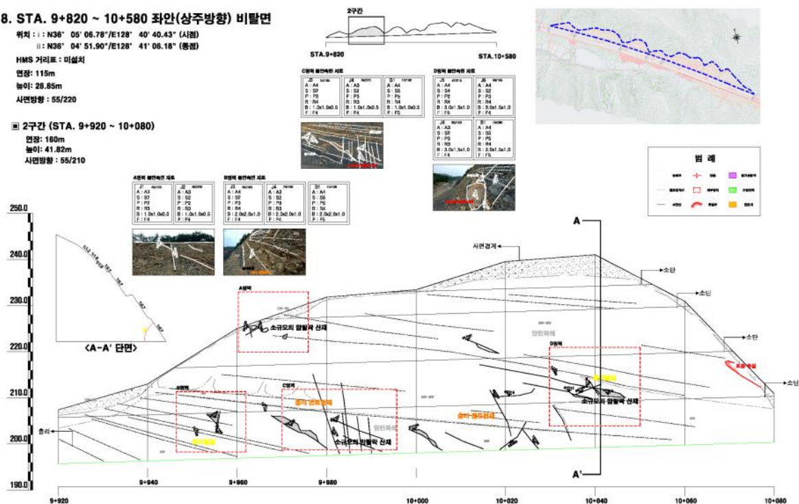
【그림 37.14】 상주절토 37 검토대상 비탈면구간
