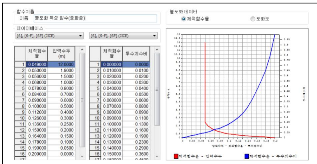
【그림 37.15】 압력수두-체적함수(포화도)-투수계수비 함수
